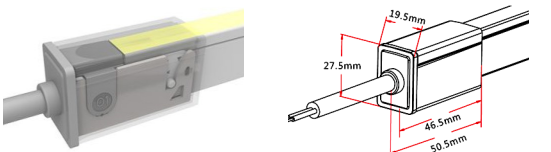
81-425 Connexion étanche IP67. Montage sur site. Sortie de câble dans l'axe. Longueur du câble 1m.
