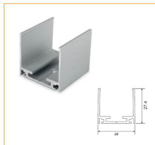
921-32-30 Clip de fixation aluminium longueur 3cm
