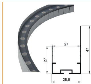
921-35-1000 Profilé inox cintrable avec rebord pour une fixation murale longueur 1m
