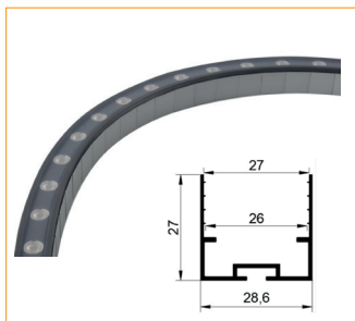
921-34-1000 Profilé inox cintrable longueur 1m
